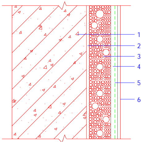
图6.2.1 保温浆料系统
