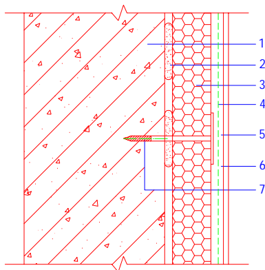
图6.1.1 EPS 板薄抹灰系统
