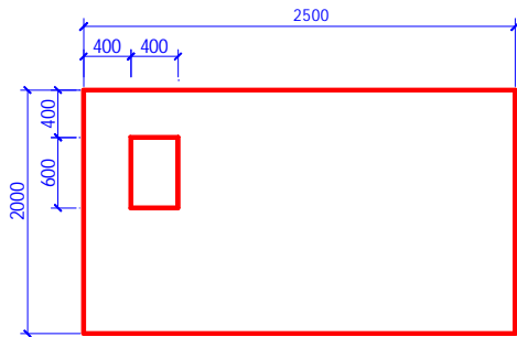
图 A.2.1 试样
