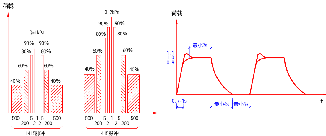
图 A. 3. 3 加压步骤及压力脉冲图形
