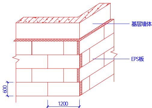
图 6.1.9 (a) EPS 板排板图
