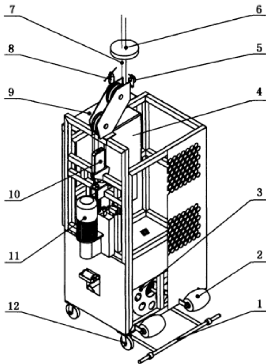
图 2 双吊点平台
