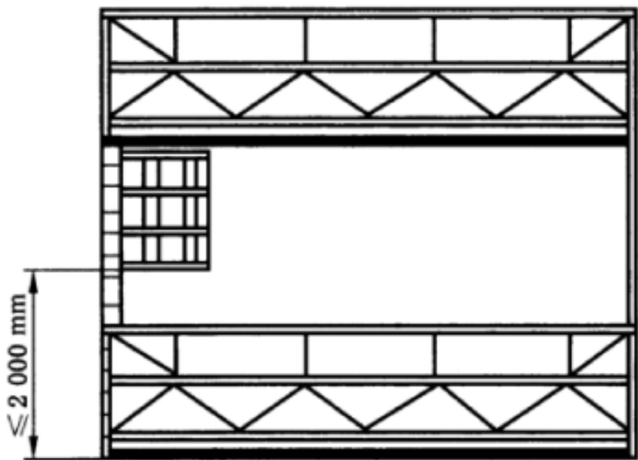
图 14 多层平台
