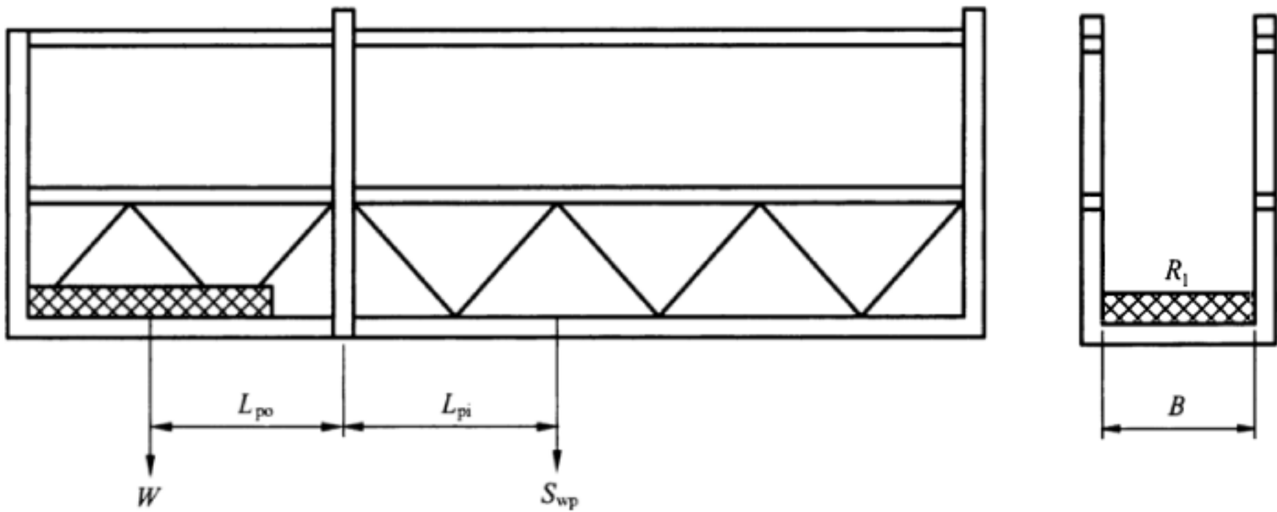
图 6 悬臂平台
