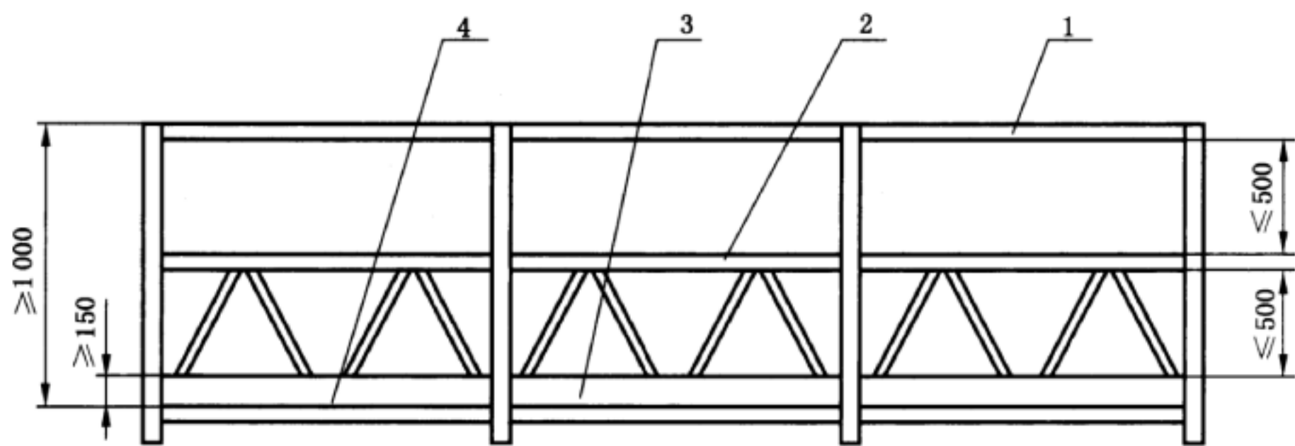
说明： 1——护栏； 2——中间护栏； 3——踢脚板； 4——平台底板。
