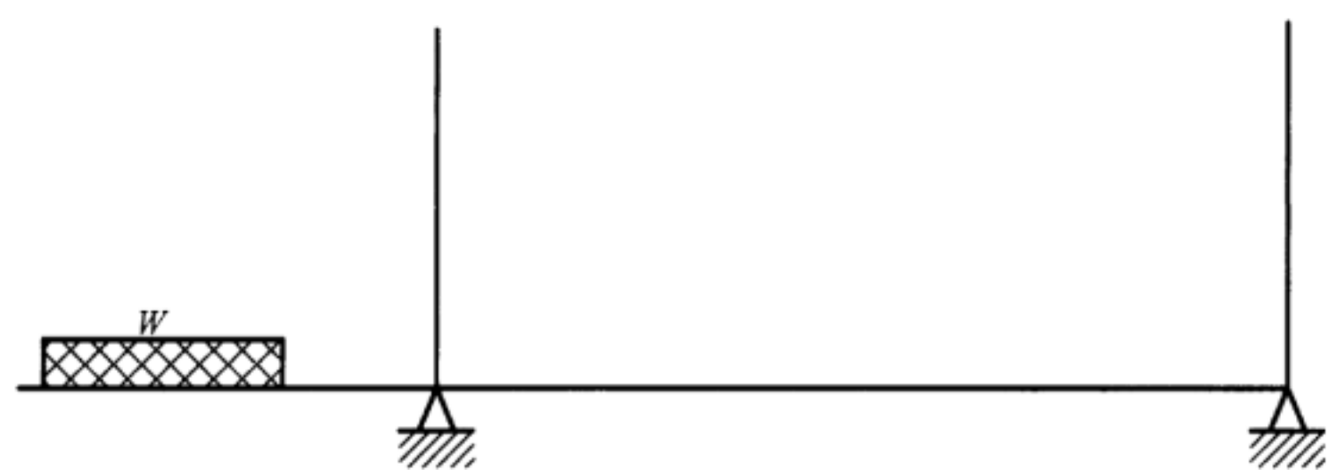
图 A.2 悬臂部分载荷
