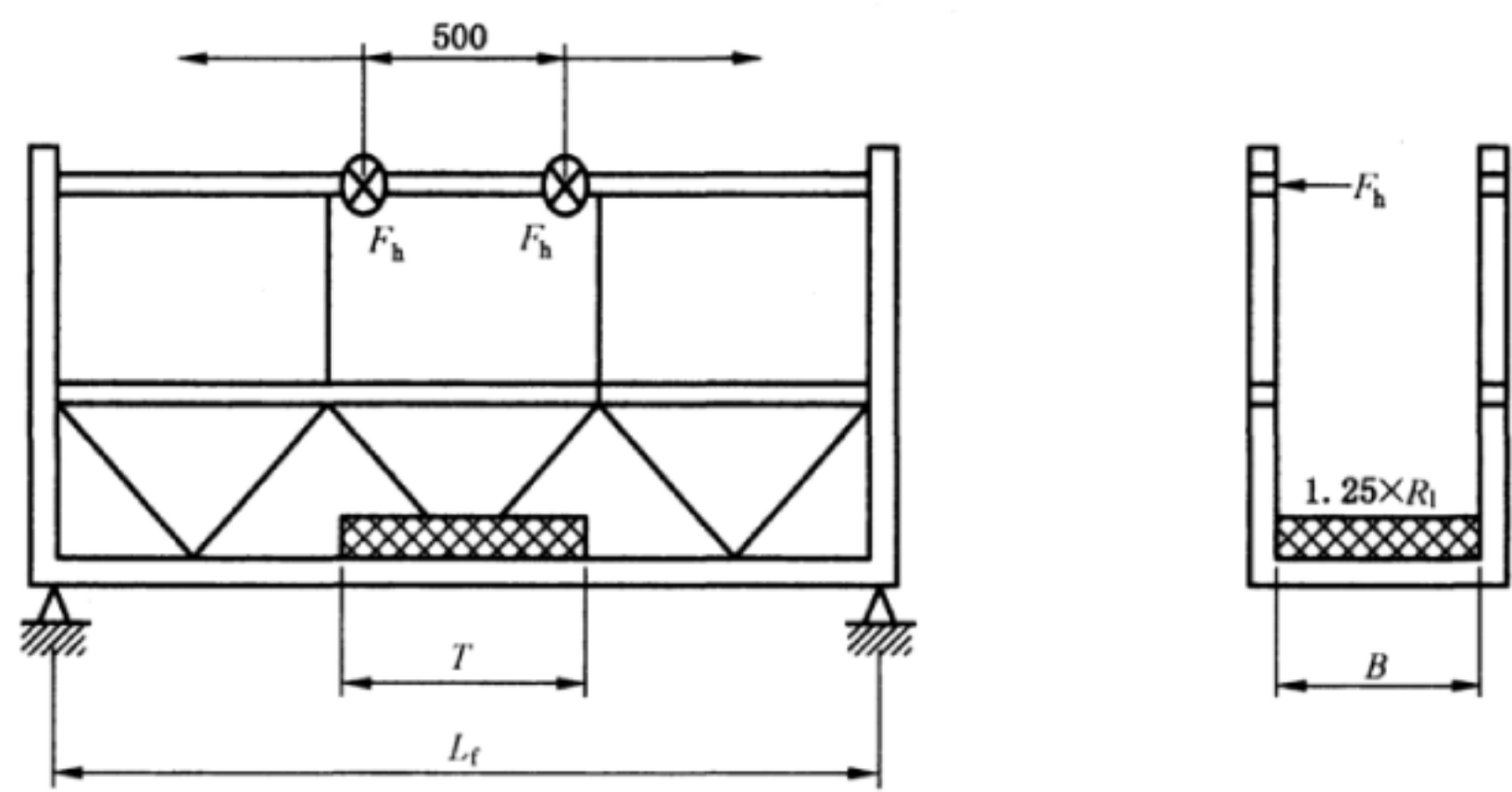
图 A.4 护栏上的水平载荷
