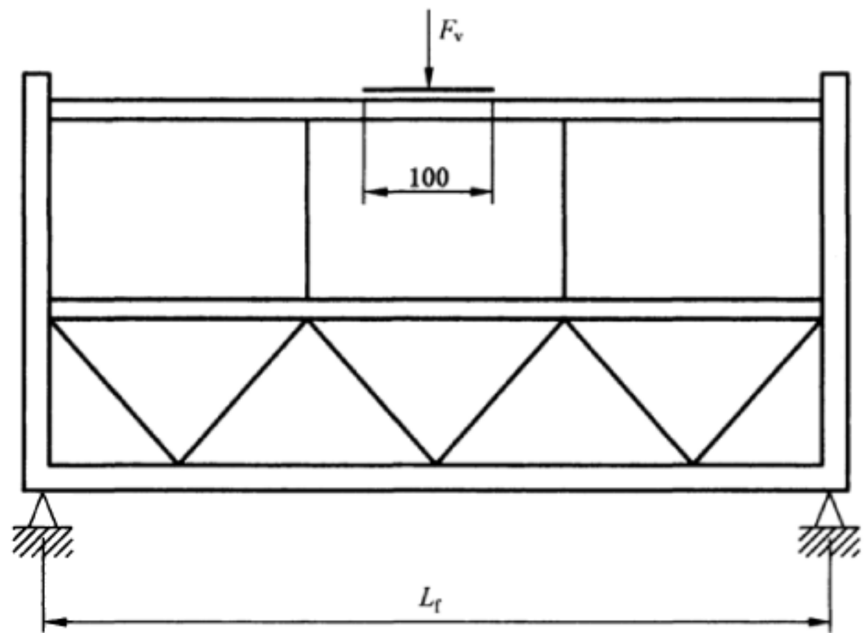
图 A.5 护栏上的垂直载荷
