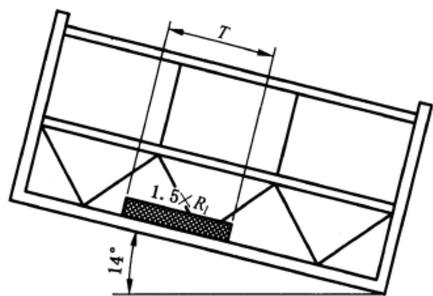
图 A.3 倾斜平台
