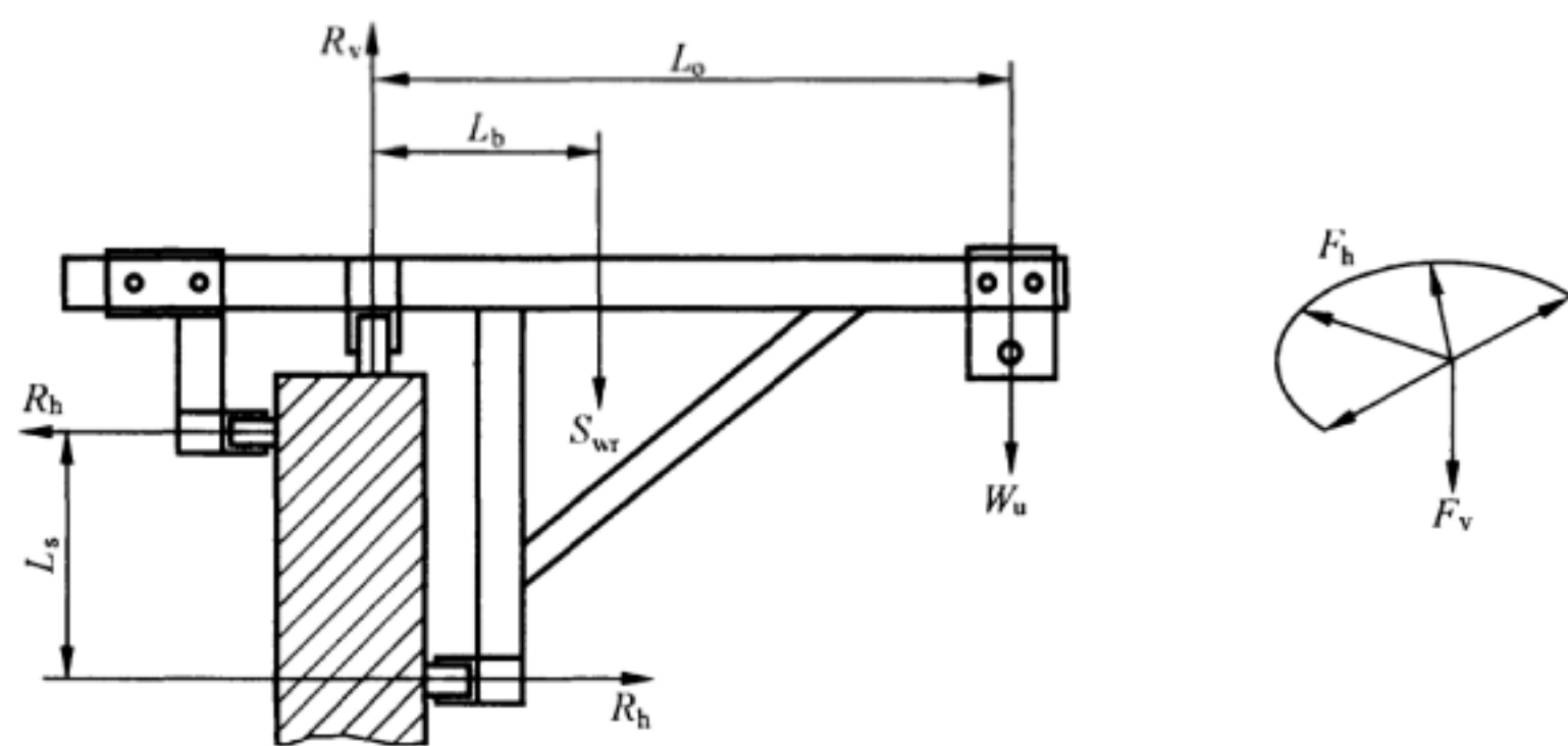
图 11 女儿墙卡钳
