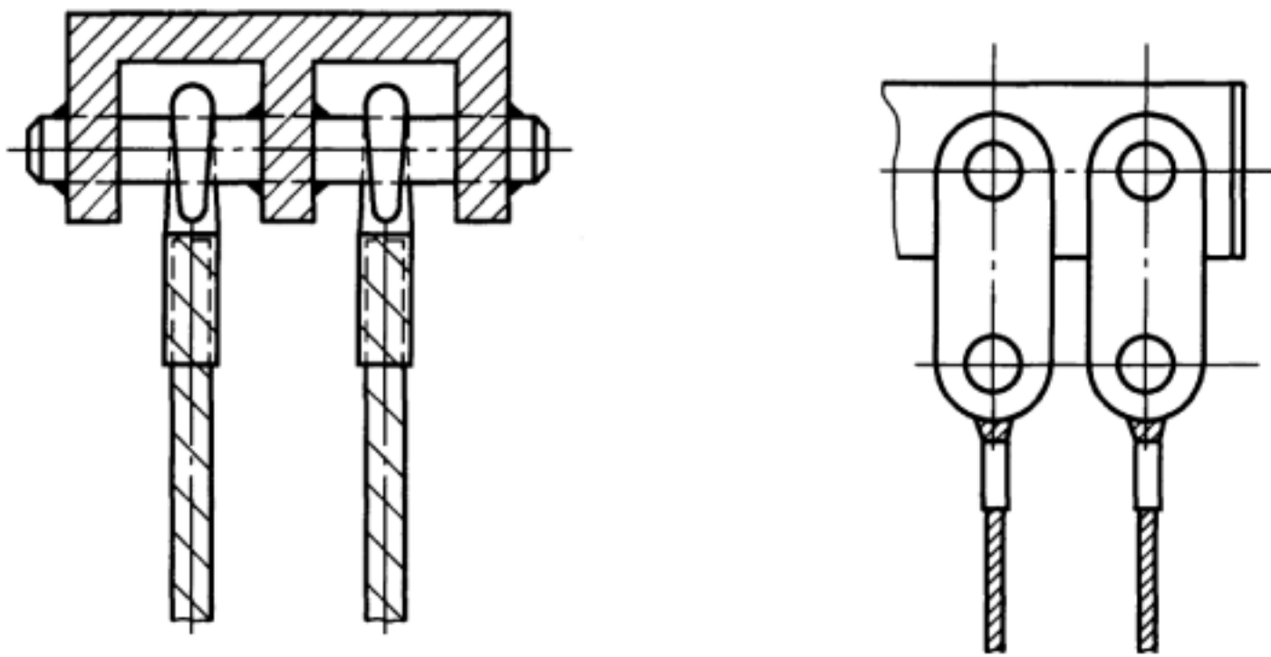
图 16 典型悬挂点示例
